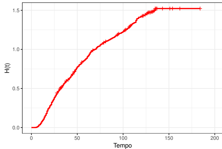
Figura 7: Função de risco acumulada Estimada.
