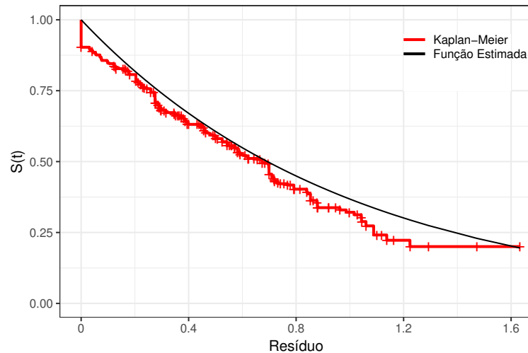
Figura 20: Resíduo de Cox-Snell.
