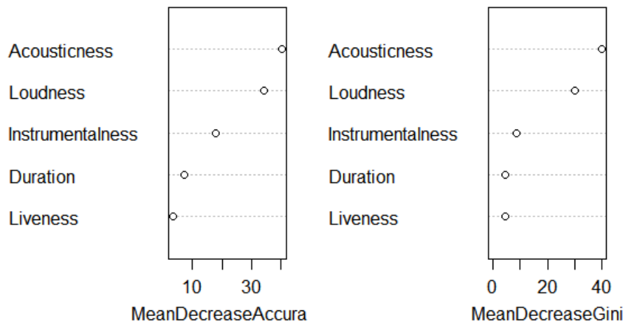
Figura 35: Importância de variáveis para o modelo 2.
