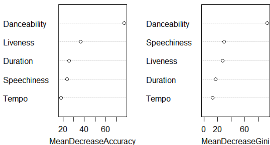
Figura 25: Importância de variáveis para o modelo 2.
