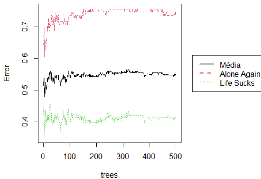
Figura 30: Erro do treino do random forest para o modelo 2.
